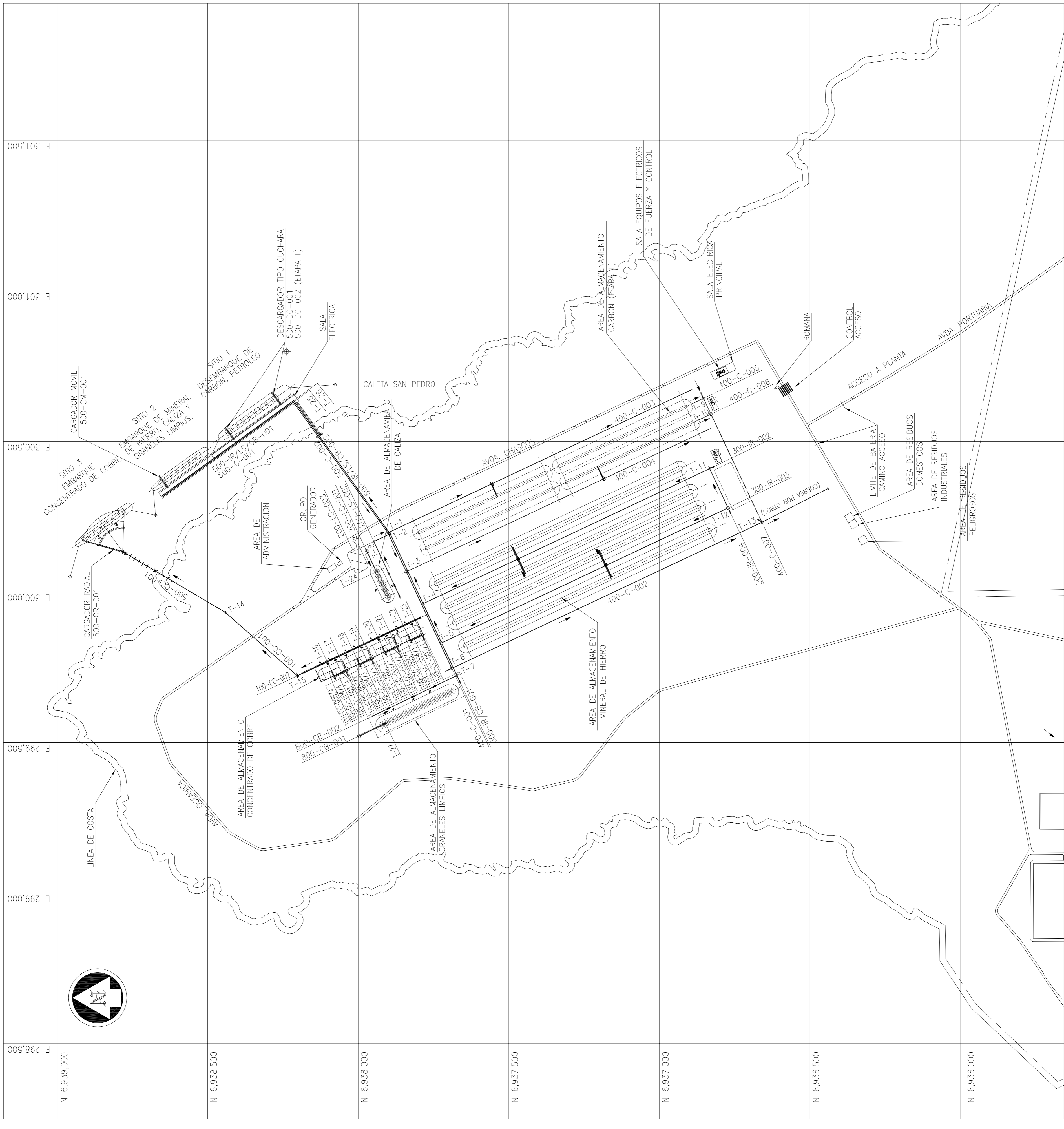
DISPOSICION GENERAL PLANTA ESC. 1:7000
